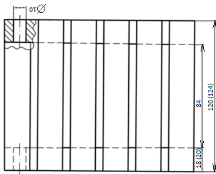
Bokorysný pohľad
